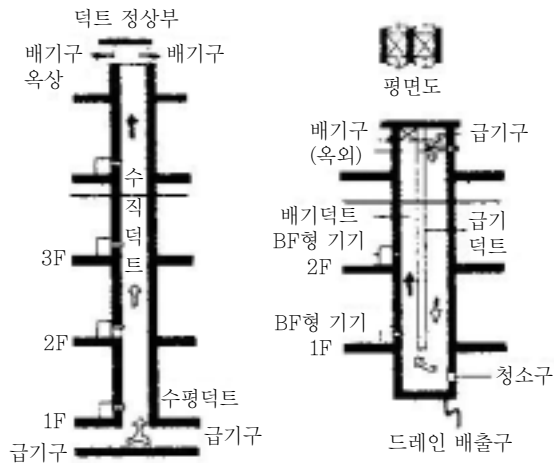
[그림 2] SE 및 U닥트의 설치 예
