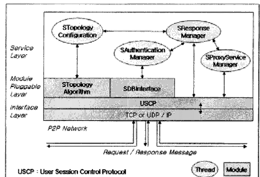
그림 2. 프록시 서버 소프트웨어 구조
