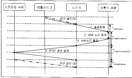
그림 10. 노드의 이탈에 따른 재배치 시간 모델
