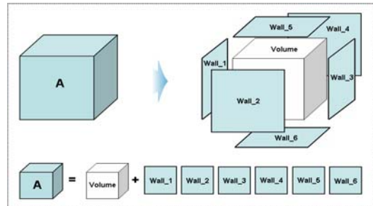
<그림 2> 3D-GIS 데이터 모델의 공간구성
