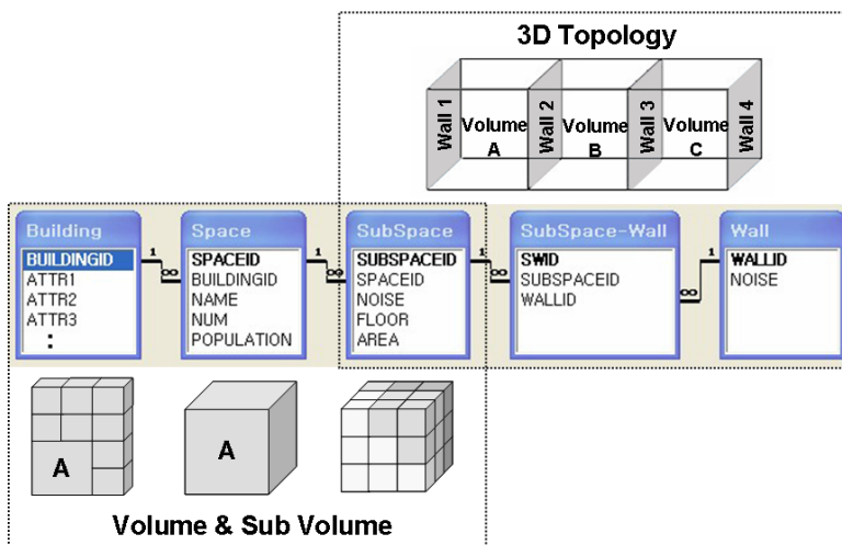
<그림 5> 데이터베이스 모델링
