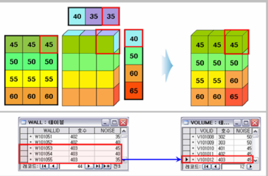
<그림 9> 볼륨데이터블에 저장되는 대표 소음값
