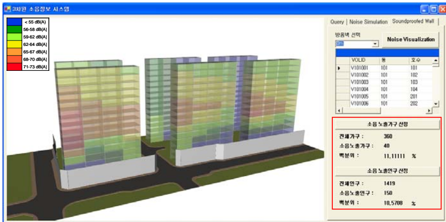
<그림 11> 3차원 공간별 소음시각화(8m의 방음벽)
