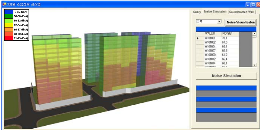
<그림 10> 시간의 변화에 따른 3차원 소음 시뮬레이션
