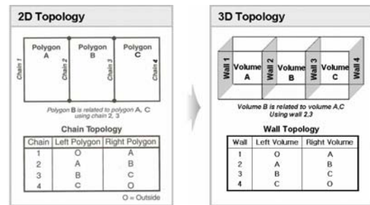
<그림 3> 2D Topology & 3D Topology
