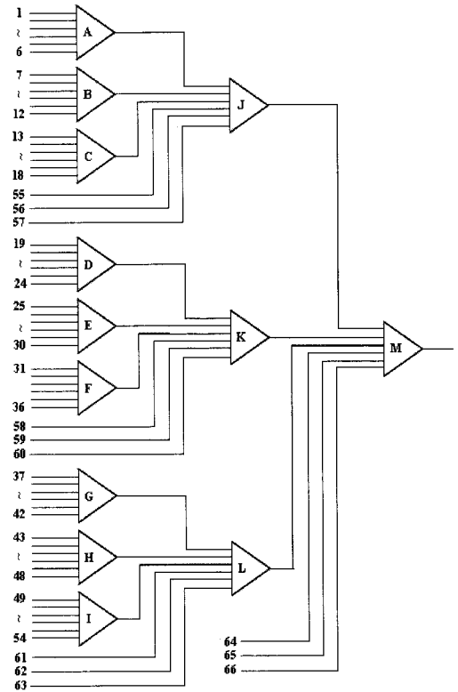
그림 5. 시뮬레이션에 사용된 다단계 비대칭형 스위치 모델
