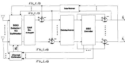
그림 14. ICI Subtractor를 적용한 Iterative-BLAST 수신단 구조
