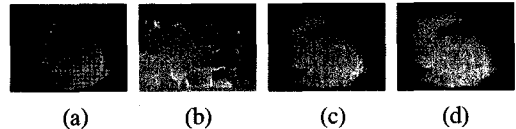
그림 2. 디지털 홀로그래프의 subsampling 후 복원 결과 (a) 원객체, (b) 1-pixel 단위 subsampling 결과영상, (c) 128×128 블록 단위의 subsampling, (d) 64×64 블록 단위의 subsampling
