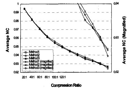
그림 17. 3D segment scanning 방식에 따른 평균 NC 결과 (회전 객체)
