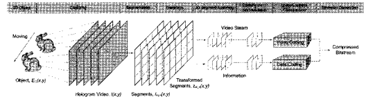
그림 6. 디지털 홀로그램 비디오 부호화
