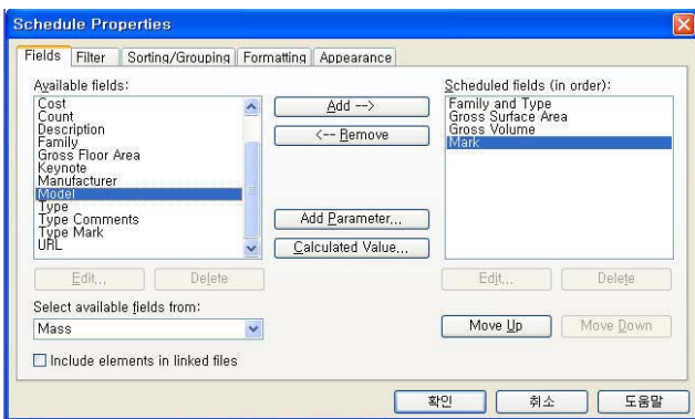
그림 12. 부문별 일람표작업화면
