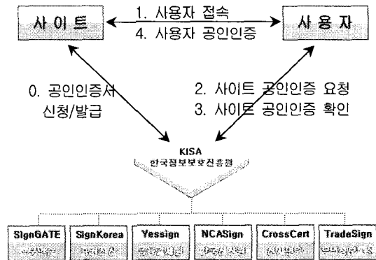
그림 11. 공인인증 사이트 확인을 위한 데이터 흐름도(2) Fig. 11. Data Flow Chart for Certified Authentication Site Confirmation (2).
