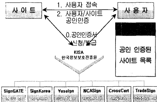
그림 9. 공인인증 사이트 확인을 위한 데이터 흐름도(1) Fig. 9. Data Flow Chart for Certified Authentication Site Confirmation (1).
