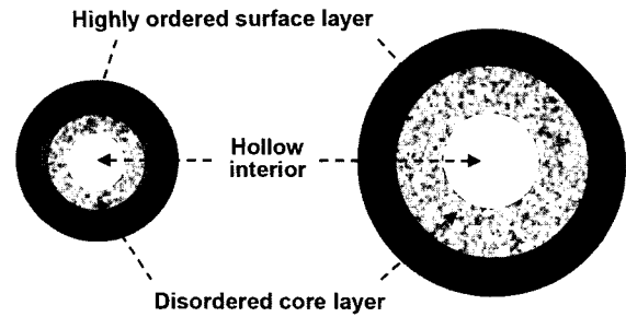
그림 7. 하드 템플레이트 기공 내에서 제조된 나노튜브의 직경에 따른 고분자 체인 규칙성의 차이를 보여주는 개략도.
