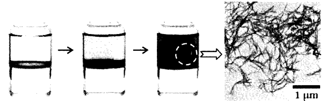
그림 5. 아닐린 단량체의 계면중합을 보여주는 사진(중합 개시 후 60초, 80초, 120초에서 촬영), 16 그리고 제조된 폴리아닐린 나노섬유의 대표적인 투과전자현미경 사진. 18
