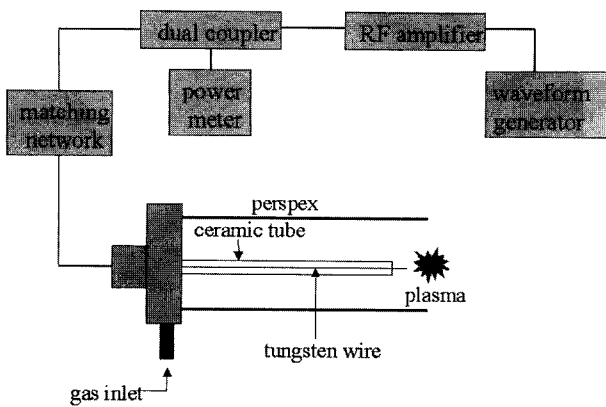
그림 1 실험 장치 개략도 Fig. 1 The schematic of experiment system
