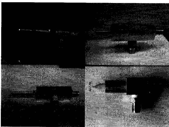
그림 2 다양한 플라즈마 발생 팁 Fig. 2 Various plasma tips tested in the experiment
