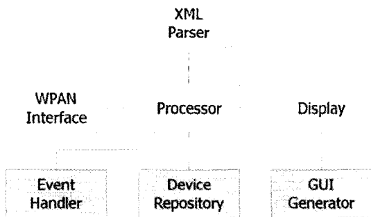
(그림 2) URC의 소프트웨어 프레임워크 구조
