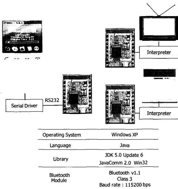
(그림 10) 시스템의 구성과 환경
