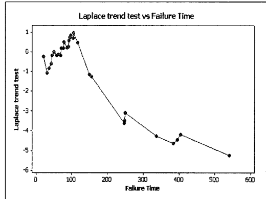
그림 2. 라플라스 추세 검정 Figure 2. Laplace trend test
