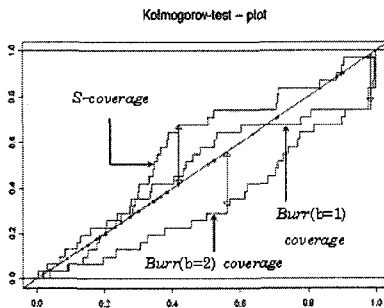
그림 3. 모형에 대한 Kolmogorov 검정 Figure 3. Kolmogorov test of each model
