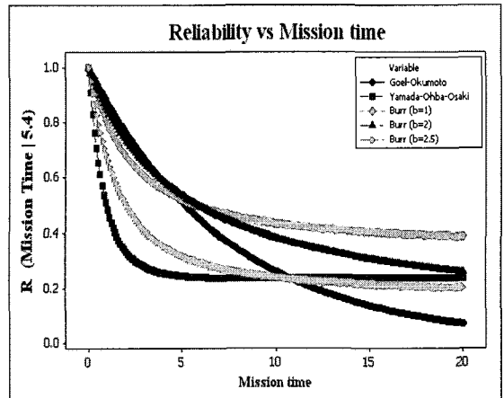
그림 6. 각 모형에 대한 신뢰도 Figure 6. Reliability of each model
