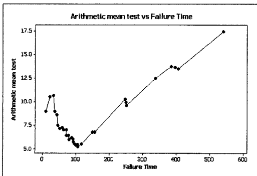
그림 1. 산술평균검정 Figure 1. Arithmetic mean test
