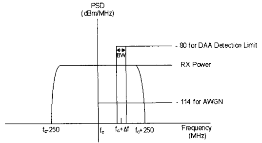
그림 10. 시뮬레이션을 위한 신호별 상대적인 전력비 Fig. 10. Relative PSD(Power Spectrum Density) ratios for simulation.
