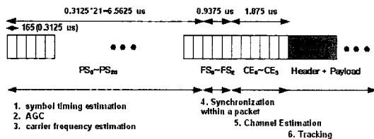
그림 7. MB-OFDM UWB system의 프리앰블 구조 Fig. 7. Preamble structure of MB-OFDM UWB system.
