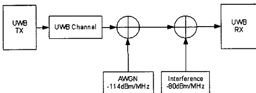
그림 9. 시뮬레이션의 간섭 구조 Fig. 9. The interference structure for simulation.
