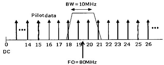
그림 11. MB-OFDM UWB system의 128 FFT 윈도우 내에서 WiMAX 간섭 신호 위치 Fig. 11. Position of WiMAX interference within 128 FFT Window of MB-OFDM UWB system.
