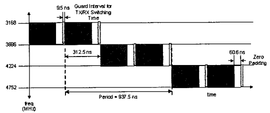
(b) TFI 모드(TFC 3) (b) TFI mode(TFC 3)
