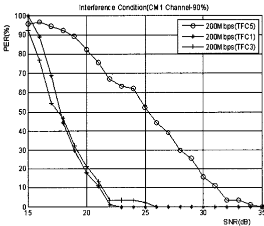
(b) CM 1 페이딩 채널 환경 (b) CM 1 fading channel environment
