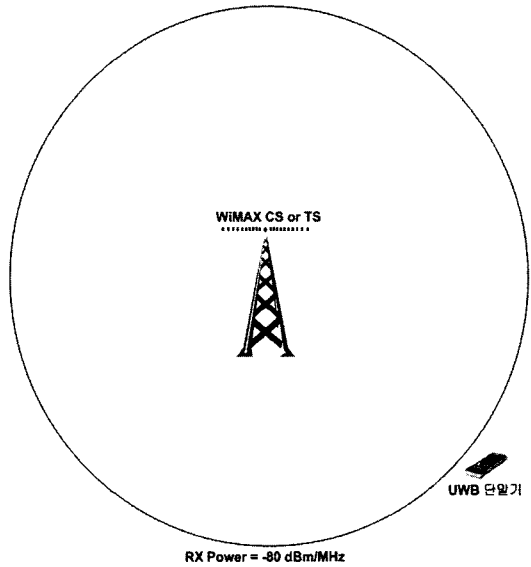
그림 6. 국내 DAA 기술 기준에 따른 UWB 단말기 회피 범위
