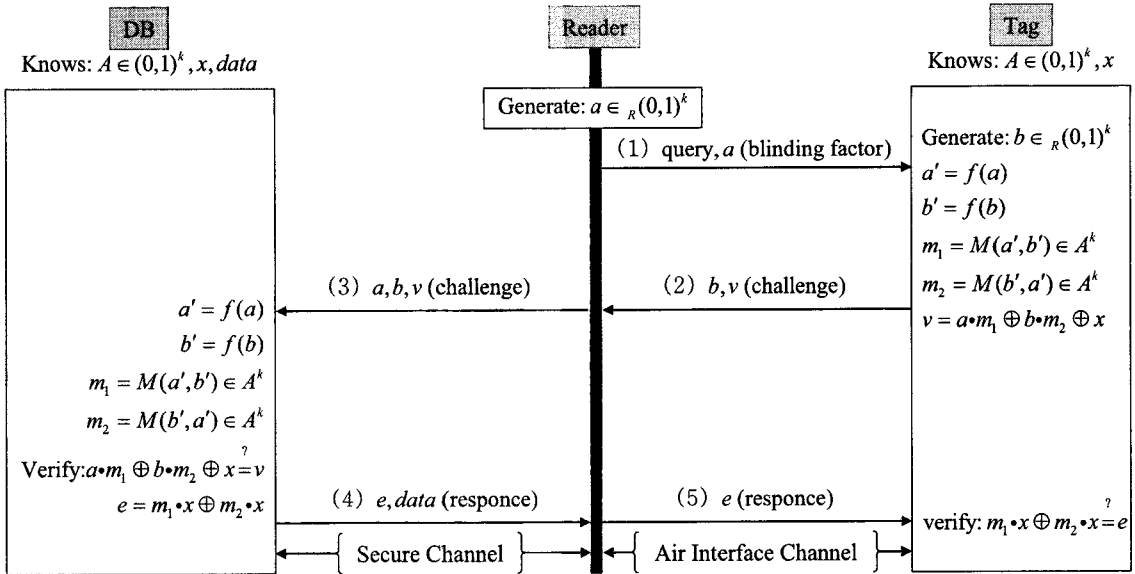
그림 2. 제안한 행렬기반 RFID 상호인증 프로토콜
