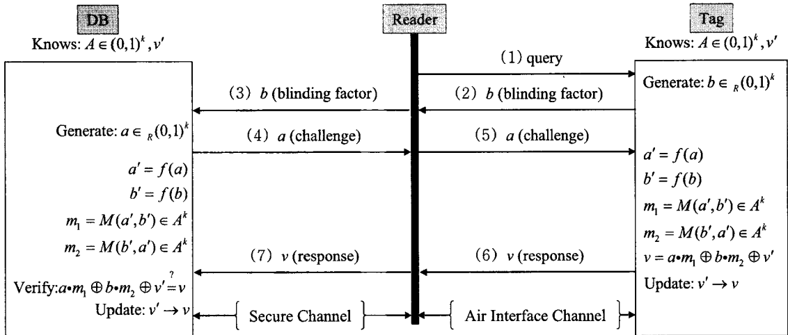
그림 1. Lee와 Ahn의 행렬기반 RFID 인증 프로토콜
