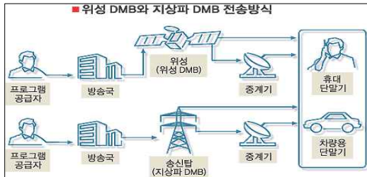
(그림 2) DMB 서비스 시스템 비교
