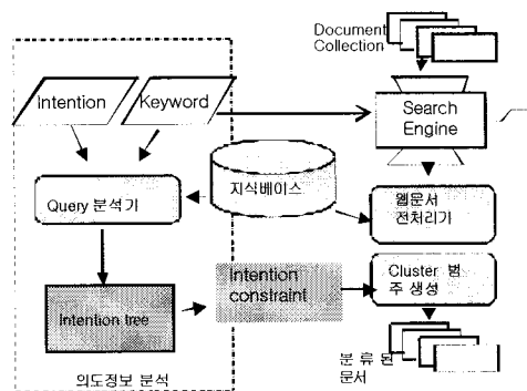
<그림 5> HDCI 구성도
