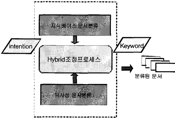
<그림 6> 하이브리드 조정 프로세스
