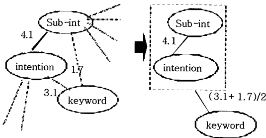
<그림 2> 병합을 통한 그룹의도와의 관계
