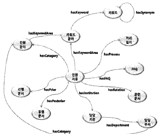
<그림 4> 의미를 고려한 온톨로지 설계 사례
