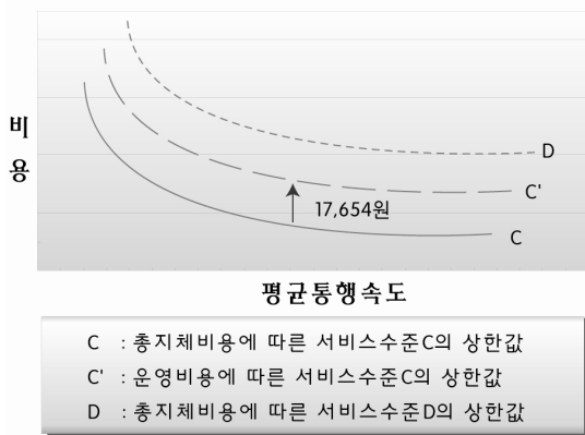
〈그림 4〉 사고비용을 고려한 경우 서비스수준의 변화
