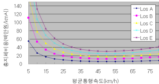
〈그림 3〉 평균통행속도와 총지체비용과의 관계
