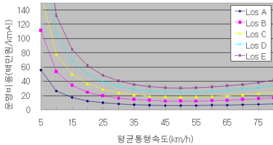
〈그림 2〉 평균통행속도와 운영비용과의 관계
