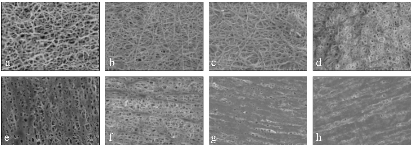
Fig. 2. 소독 후 PPDO-hybrid-PLGA scaffold의 SEM 사진 (× 1K) 외층표면(PLGA): a: 대조군, b: Alcohol, c: EO65, d: EO37 와 내층표면(PPDO): e: 대조군, f: Alcohol, g: EO65, h: EO37
