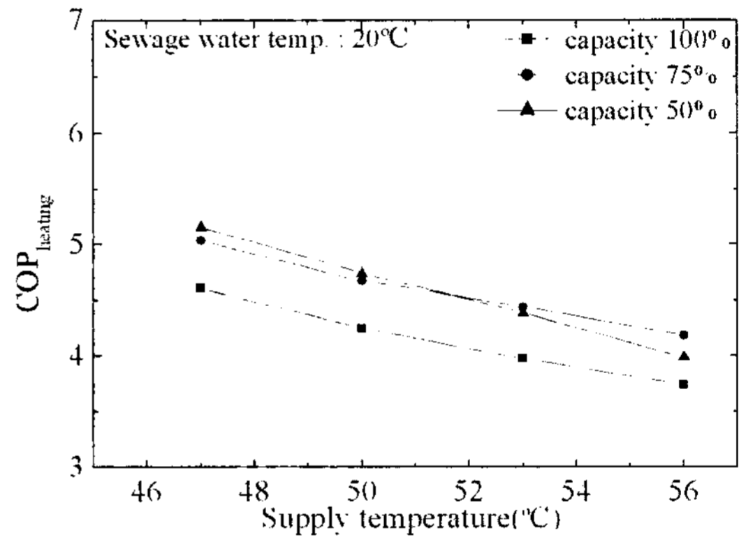
[그림 8] 공급온도에 따른 난방용량
