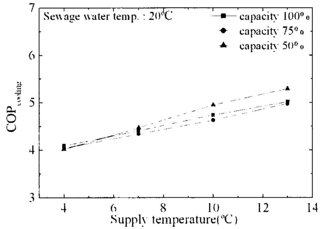
[그림 6] 공급온도에 따른 냉방 COP
