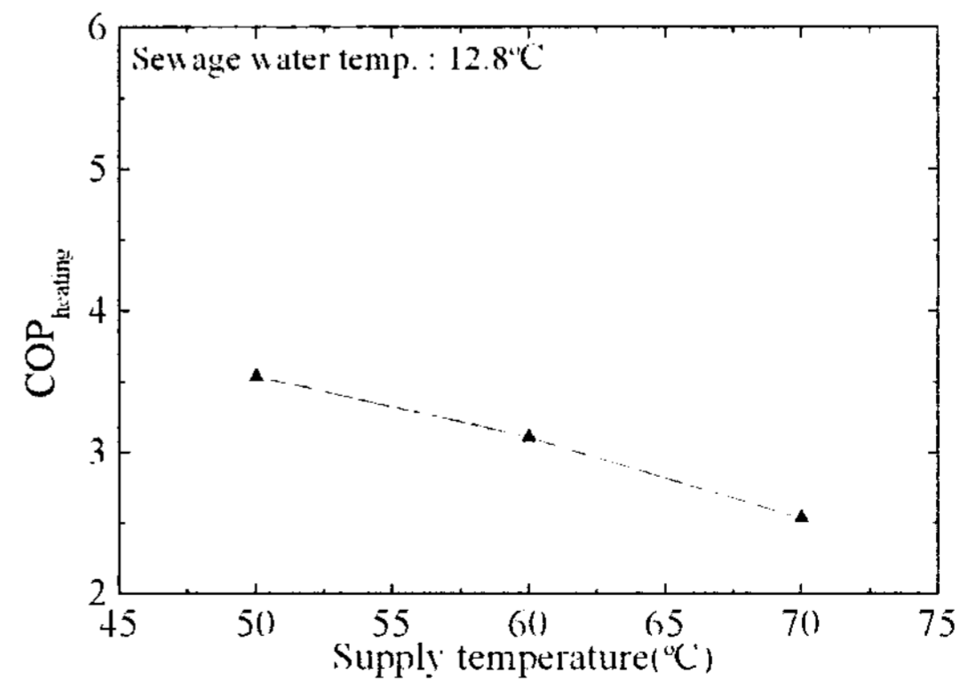
[그림 10] 공급온도에 따른 난방용량 (2단운전)
