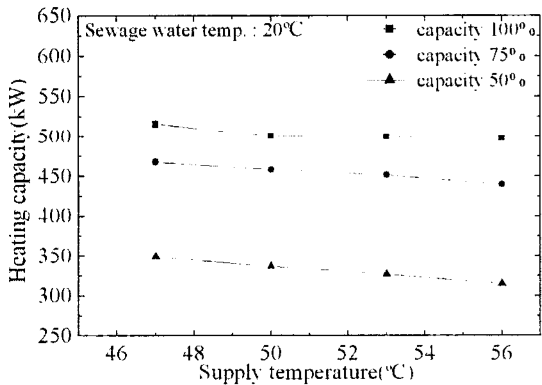
[그림 7] 공급온도에 따른 난방용량
