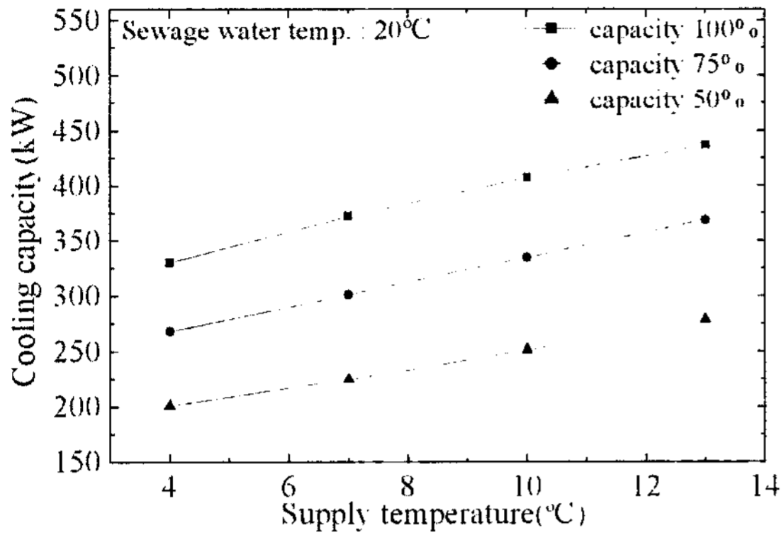
[그림 5] 공급온도에 따른 냉방용량
