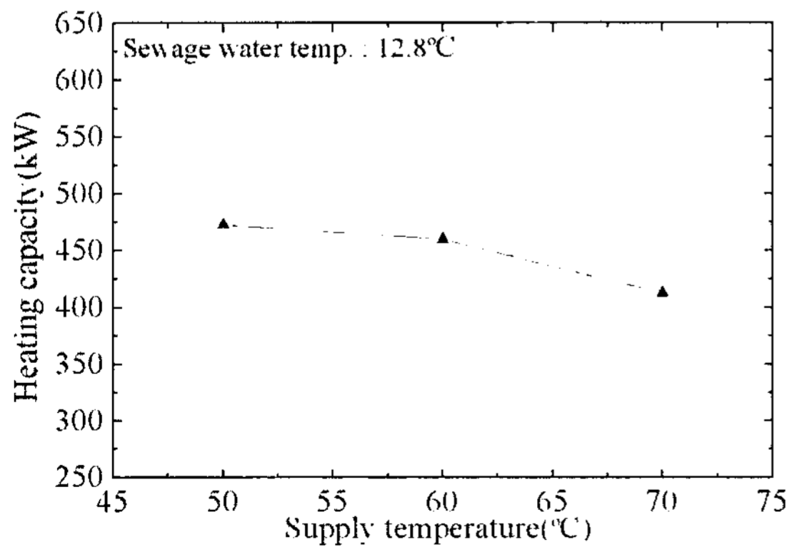
[그림 9] 공급온도에 따른 난방용량 (2단운전)
