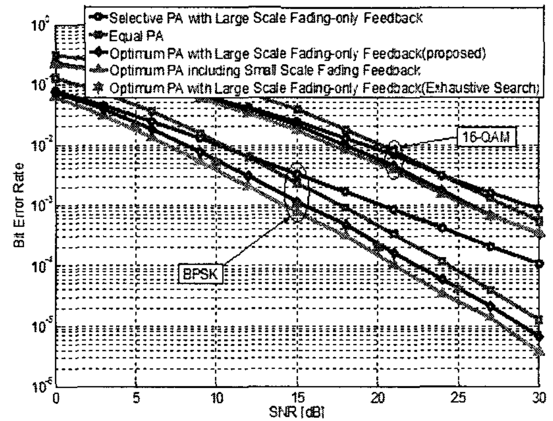
그림 2. 전력 분배 기법들에 따른 평균 BPSK와 16-QAM BER 성능 비교, \alpha=4, \sigma_\zeta=12, \beta=1 인 Rayleigh Fading Channel.
