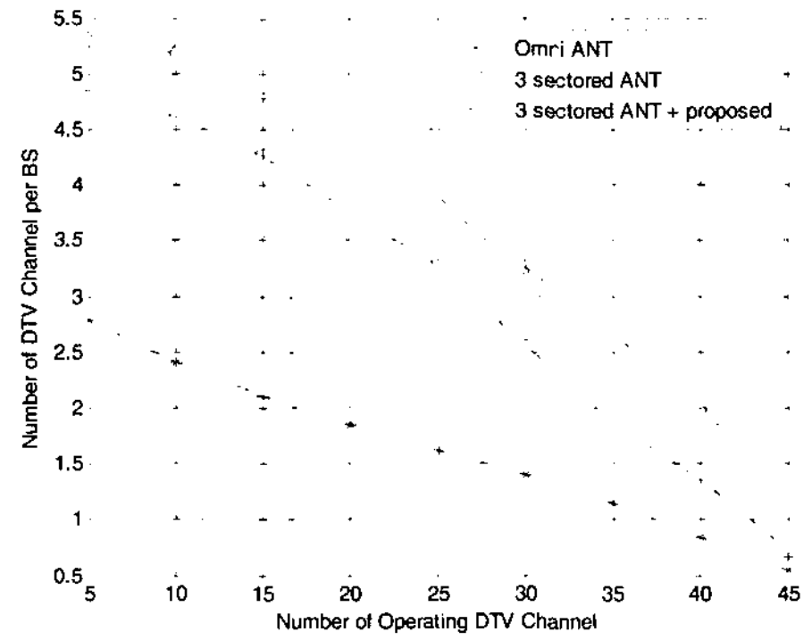
그림 3. BS당 할당된 TV 평균 채널 개수
