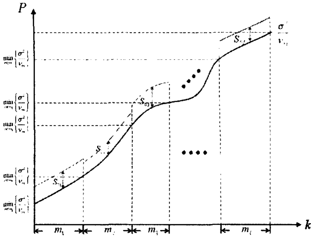
그림 2. Partial Constant Power Water-filling
