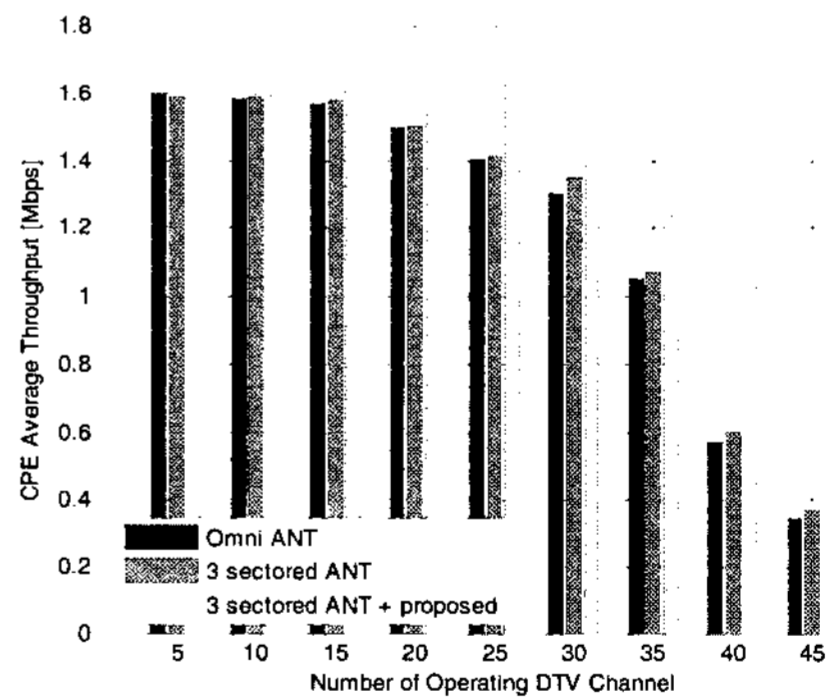
그림 7. 할당 알고리즘을 적용한 평균 CPE의 처리율
