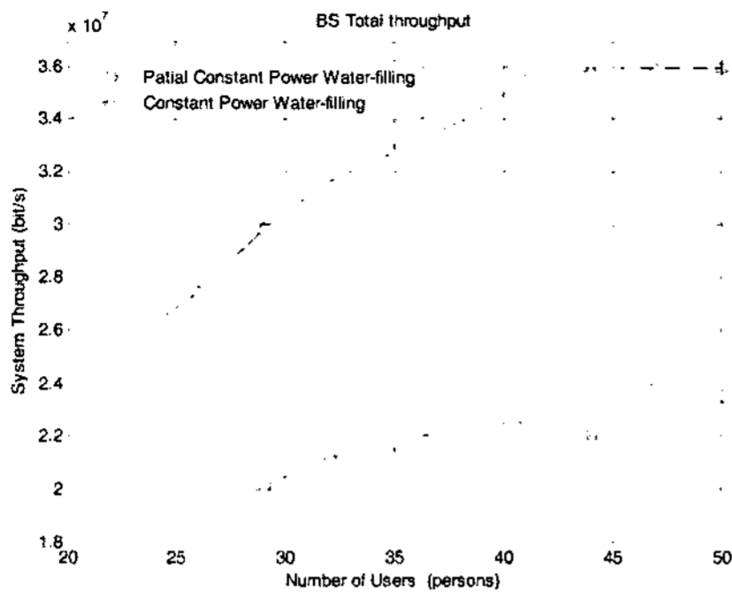
그림 5. 셀 내의 사용자 수 별 데이터 처리율
