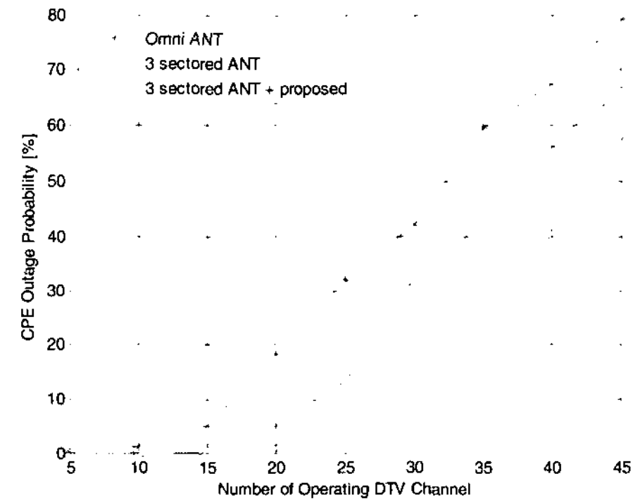
그림 4. CPE outage 확률
