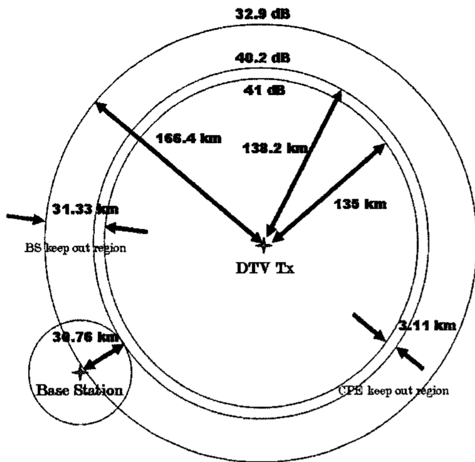
그림 1. 간섭 방지 구역의 예 [3]
