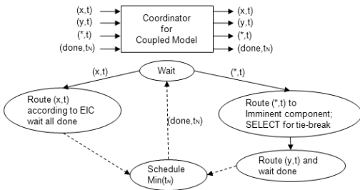
그림 3. 코디네이터 알고리즘
