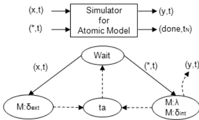
그림 2. 시뮬레이터 알고리즘
