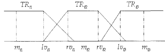
그림 1. 퍼지 패턴을 표현하는 소속함수
