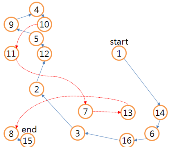
(그림 8) MaxCoverage 알고리즘에 의한 방문 순서도
