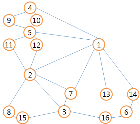
(그림 7) 분할된 그리드 맵에 대한 그래프
