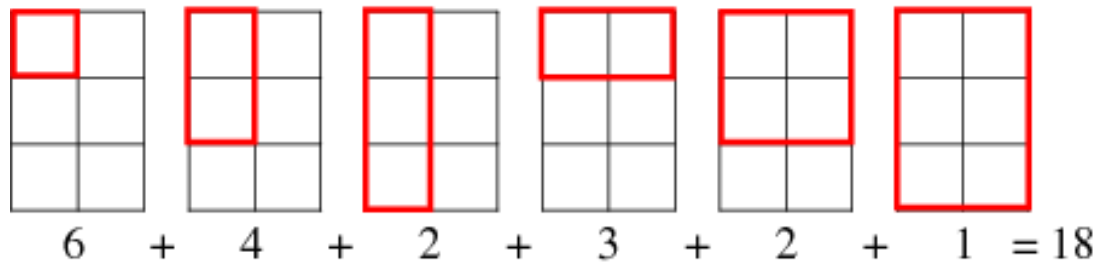
(그림 3) Rectangle Tiling 예제(출처: http://mathworld.wolfram.com/RectangleTiling.html )
