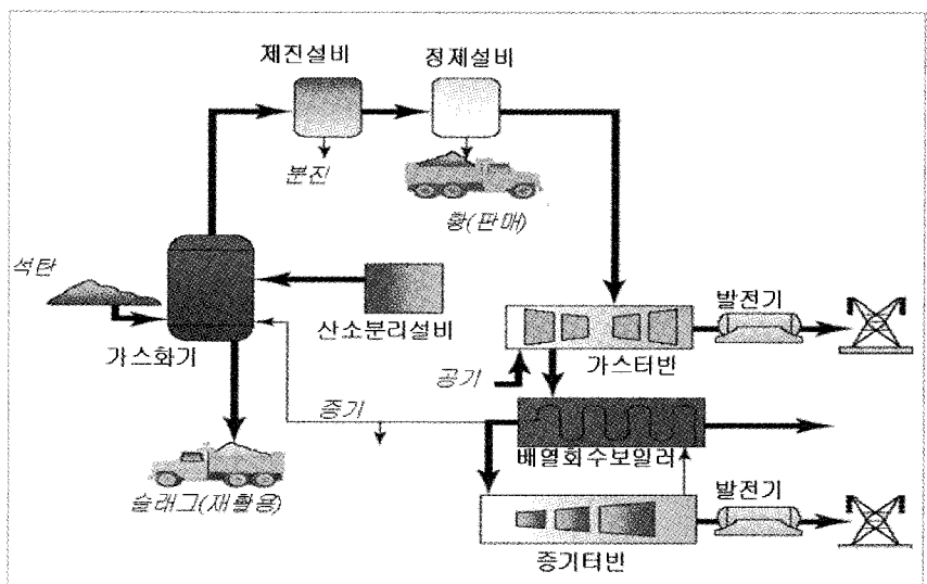
그림 1 IGCC의 구성도
