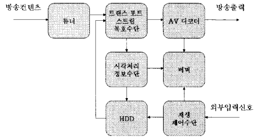
그림 2. Time-Shift 시스템 블록도(4) Fig 2. Time-Shift System Block Diagram(4)
