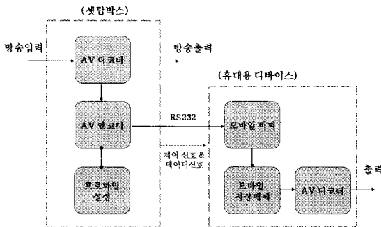
그림 3. 휴대용 멀티미디어 디바이스 TPO-Shift 블록도 Fig 3. TPO-Shift Block Diagram for Mobile Multimedia Devices
