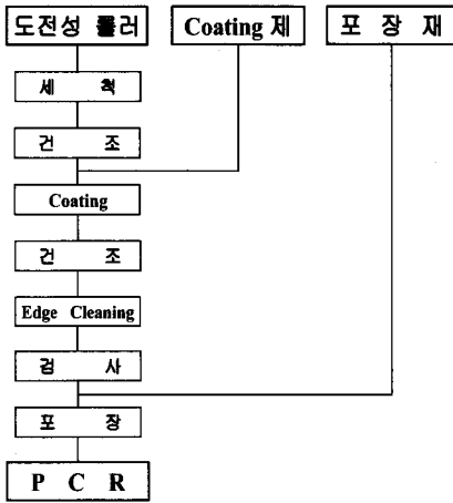
[그림 5] 대전 롤러의 제조 공정
