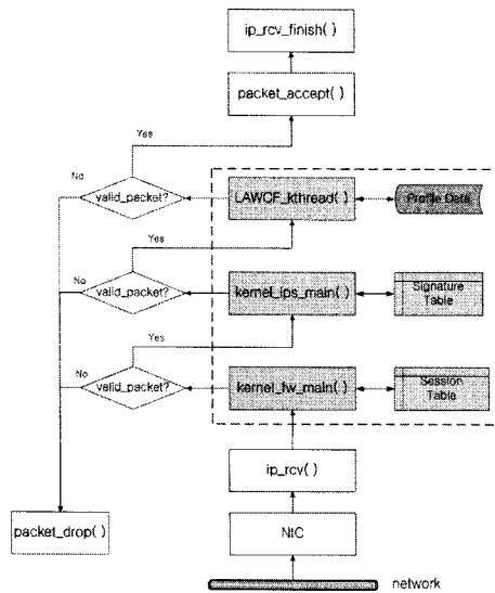
그림 2. 커널 수준에서 패킷 처리 흐름도 fig. 2. Packet Processing Flow Chart in Kernel Level
