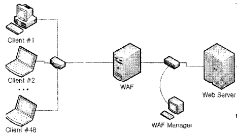
그림 6. 실험 1 환경 fig. 6. Environment of Experimentation 1
