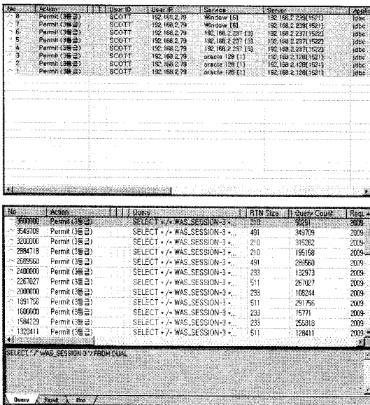
그림 19. 개선된 방식 테스트 결과 Fig 19. Improvement method test result
