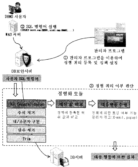
그림 16. 정형 쿼리 탐지 과정 Fig 16. Fixed form query detection process
