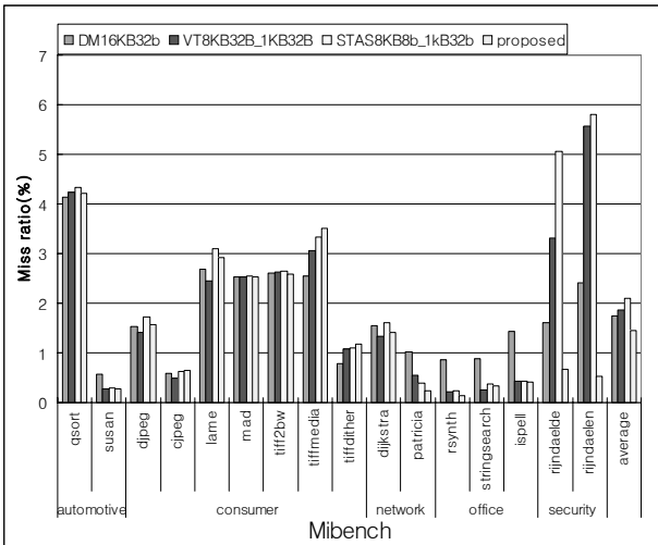
(그림 4) Mibench : 메모리 접근 실패율
