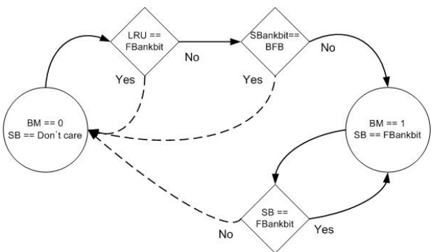
(그림 2) 제안된 상태 비트의 흐름도
