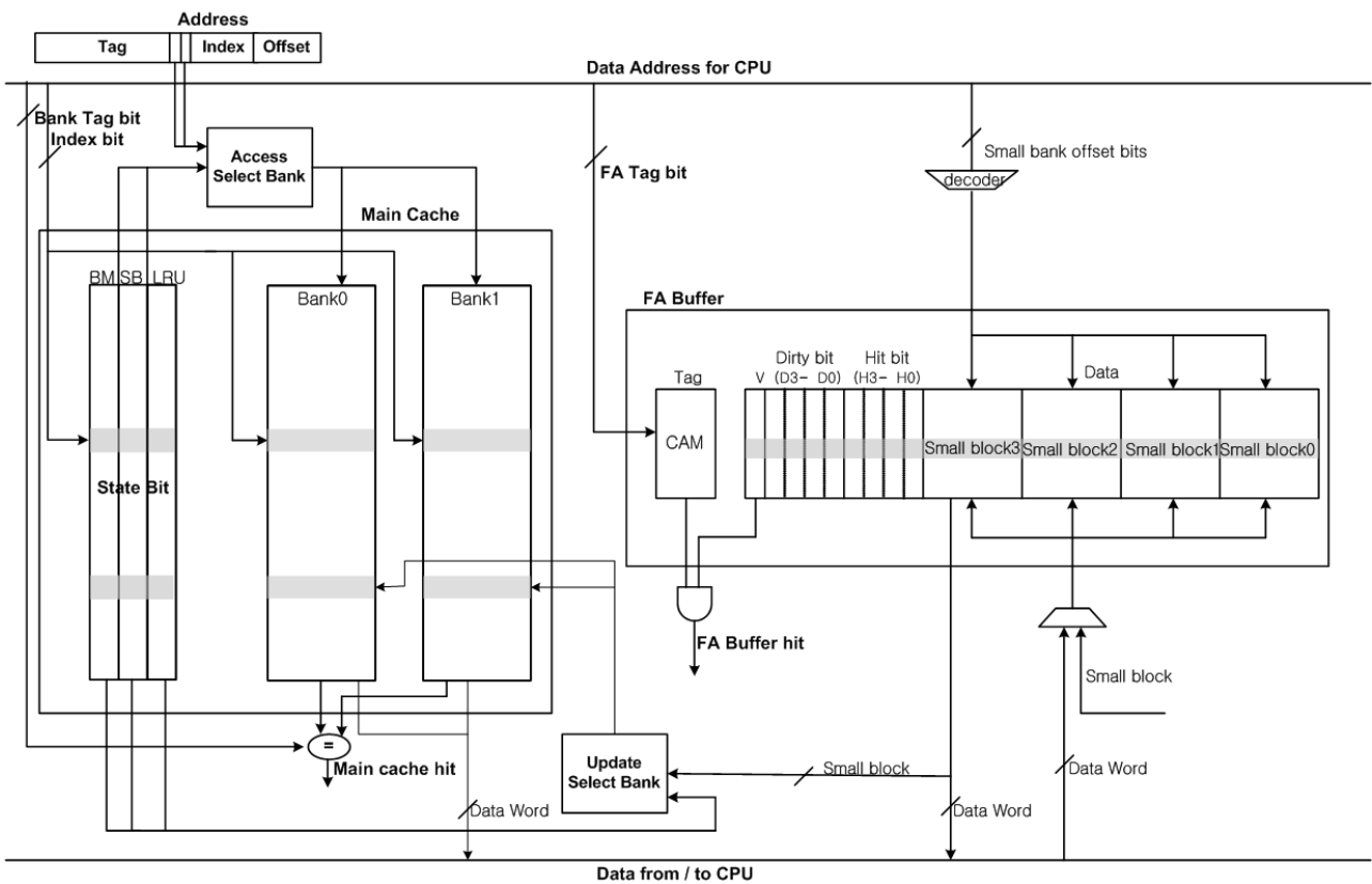
(그림 1) 제안된 캐쉬 시스템 구조
