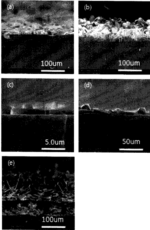
그림 2. TMSP-TBA로 표면개질된 Si 웨이퍼 위에 성장된 MFI membrane의 FESEM 단면 이미지 (a) 중력대방향, 175 °C 성장 (b) 중력방향, 175 °C 성장 (c) 중력반대, 120 °C 성장 (d) 중력반대, 140 °C (d) 표면개질 안 된 웨이퍼, 중력 반대방향 성장, 175 °C.
