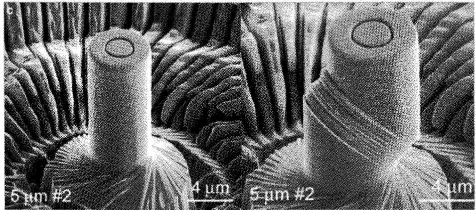
그림 2 마이크로 압축 시험의 대표적인 결과 사례; 시험 전 (왼쪽) 및 시험 후 (오른쪽), Acta Mat. (53) 4065에서 인용
