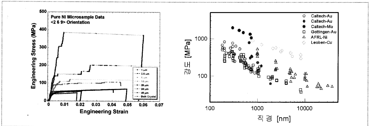
그림 3 외국 주요 연구기관의 마이크로 압축 시험 결과(왼쪽 그림은 Acta Mat. (53) 4065에서 인용, 오른쪽은 저자가 재구성)
