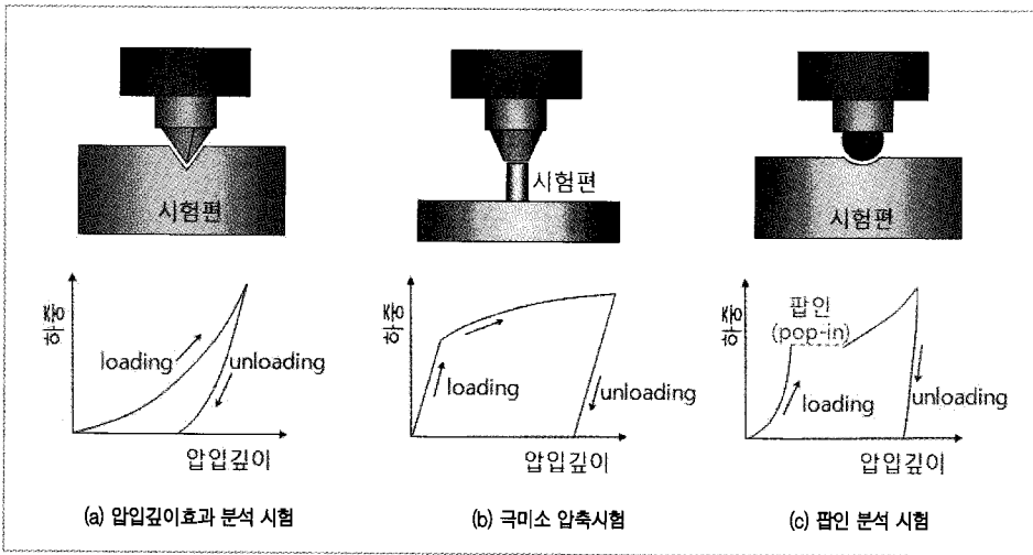
그림 1 나노 압입시험 장비를 이용한 미소 변형 거동 연구의 대표적인 사례들
