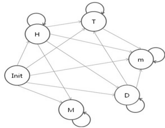
(그림 9) 연속 캐싱을 사용하는 트랜스코딩 프록시에서 D 이벤트를 추가한 이벤트 전이 그래프
