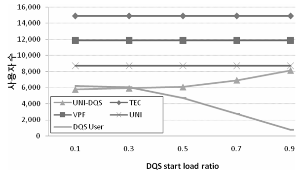
(그림 14) DQS 정책 시작 부하에 따른 지터 과발생 사용자 수
