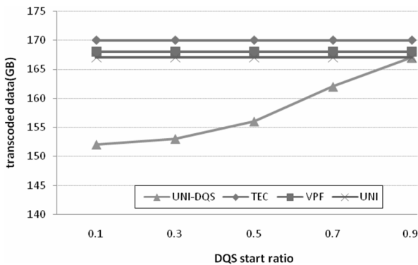
(그림 13) DQS 정책 시작 부하에 따른 트랜스코딩된 데이터 양 하가 적을 때부터 시작하게 되면 그 양을 월등히 줄일 수 있다.
