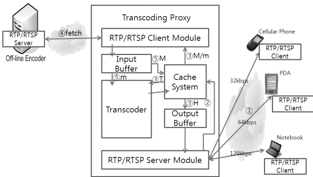
(그림 2) 트랜스코딩 프록시의 구조
