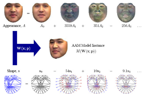
(그림 2) AAM의 shape 및 appearance model [20]
