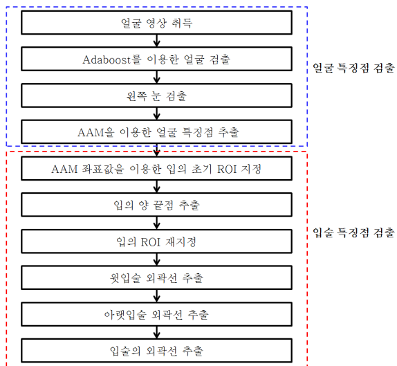
(그림 3) 제안하는 방법의 전체 흐름도
