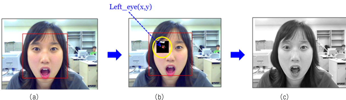
(그림 4) AAM 초기 값 설정과정: (a) Adaboost를 이용하여 얼굴 영역 검출 (b) 검출 영역 내에서 영상처리를 통한 이진화 및 컴포넌트 라벨링을 통한 왼쪽 눈 검출 (c)왼쪽 눈 좌표기반 AAM 특징점 검출
