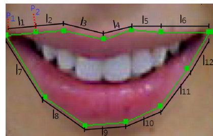
(그림 14) 실제 입술의 ground-truth 좌표 값 (녹색 및 녹색 사각 점)
