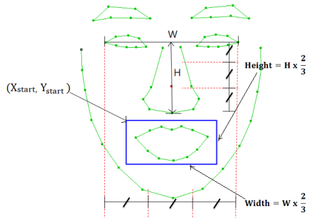
(그림 5) 얼굴의 영역별 비율에 따른 초기 관심 영역 지정
