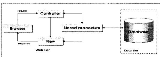
그림 3. 개발 프레임워크 동작원리 Fig. 3. Running Mechanism
