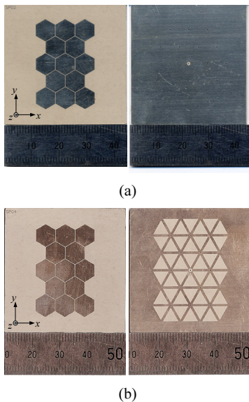
[그림 5] (a) 슬롯이 없는 안테나의 제작 사진과 (b) 슬롯 접지면이 적용된 안테나 제작 사진
