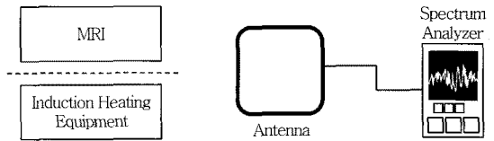
(그림 7) 측정구성도
