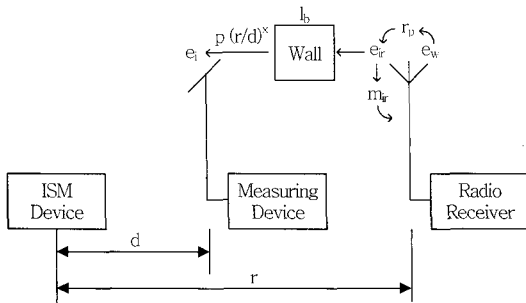
(그림 1) ISM 기기의 기준치 계산을 위한 기본모델
