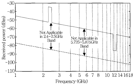
(그림 6) 1~18GHz 사이 Group 2/Class B의 수신전력
