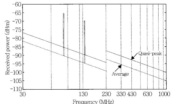
(그림 5) 30MHz~1GHz 사이 Group 2/Class B의 수신전력
