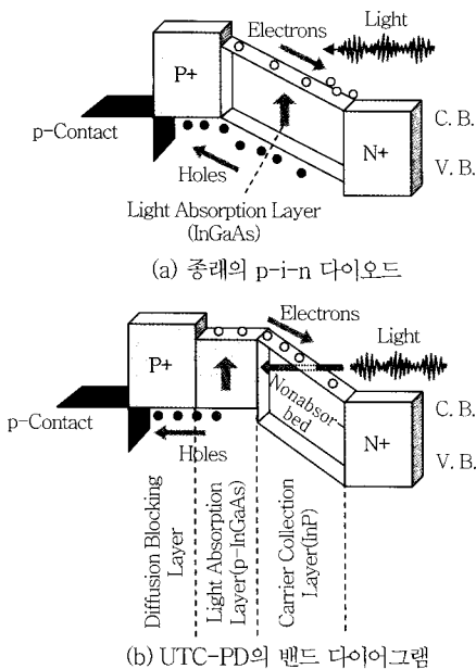
(그림 5) P-i-n PD와 UTC-PD 밴드 다이어그램
