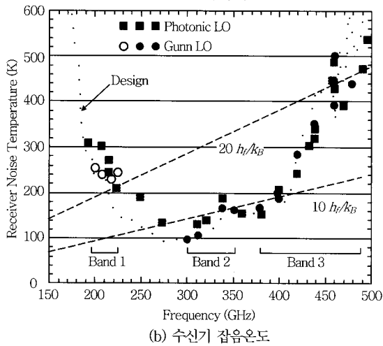
(그림 11) 광 LO와 함께 SIS 믹서를 사용한 밀리미터/테라헤르츠-파 수신기
