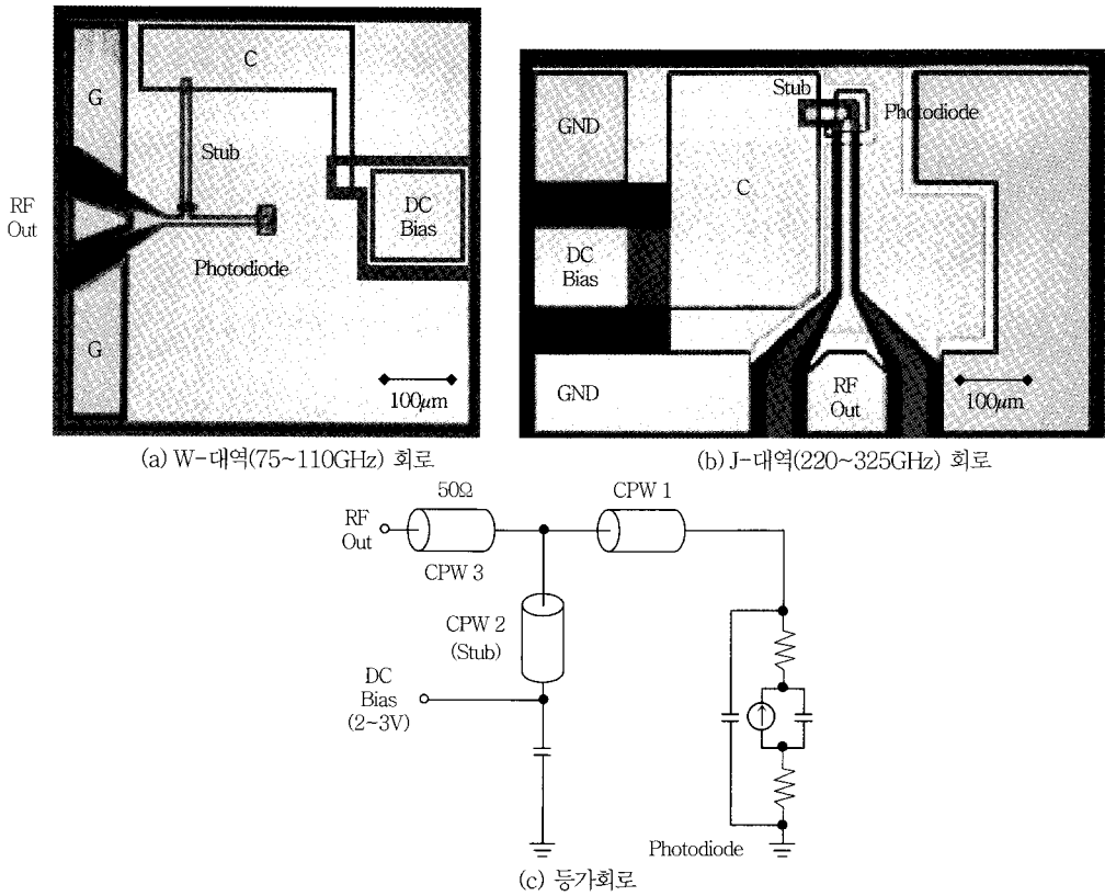
(그림 8) PD의 출력개선을 위한 회로기술
