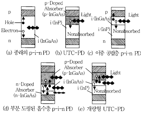
(그림 7) PD의 적층구조
