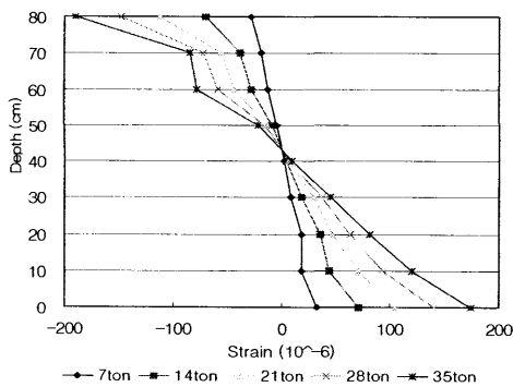
<그림 7> 중앙단면의 중립축 거동 (1회)
