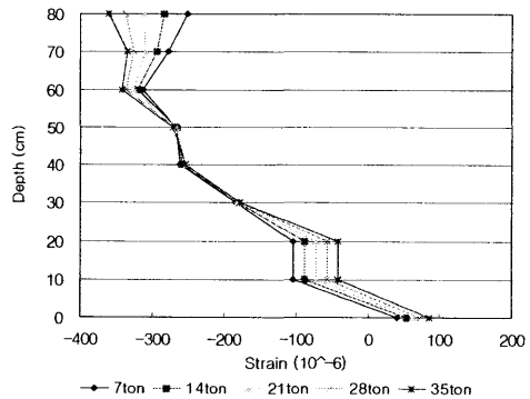
<그림 8> 중앙단면의 중립축 거동(2백만회)
