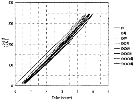
<그림 5> 중앙단면에서의 하중-변위 관계
