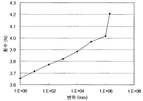
<그림 4> 중앙단면에서의 변위-반복회수
