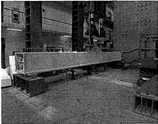
<그림 2> 피로시험체 및 가력프레임
