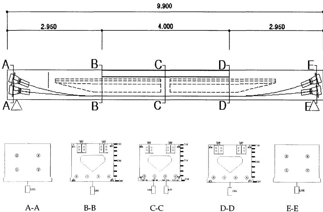
<그림 1> IT거더 시험체 제원 및 게이지 부착 위치
