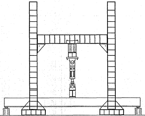
<그림 2> 피로시험체 및 가력프레임
