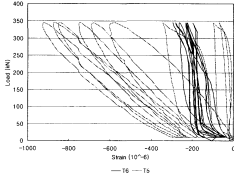
<그림 6> 1/4단면에서의 H형 강재의 변형률
