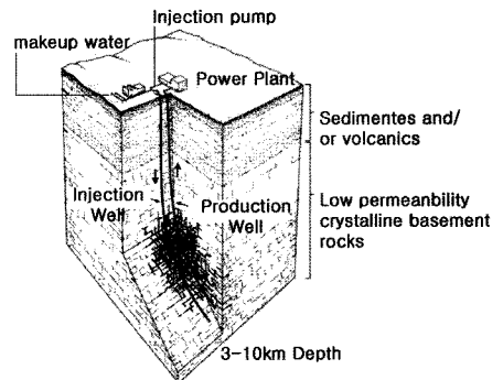
[그림 9] 복수 보어홀을 이용한 EGS 기술 개략도
