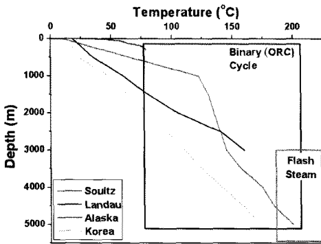
[그림 10] 국내외 주요지역의 지열구배
