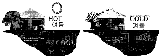
[그림 1] 지열 냉난방 시스템의 개요
