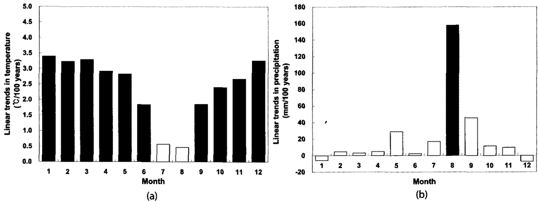
Figure 3. Linear trends of monthly average surface air temperature ( ^{\circ}\text{C}/100 years) (a) and monthly total precipitation ( \text{mm}/100 years) (b) over the last 100 years (1907-2008) in Seoul. Black bars are statistically significant at the 95% level, while white bars is not statistically significant. 지난 100년(1908~2007) 동안의 서울의 월 평균 기온( ^{\circ}\text{C}/100 년)(a)과 월 총 강수량( \text{mm}/100 년)(b)의 일차 추세 변화를.
