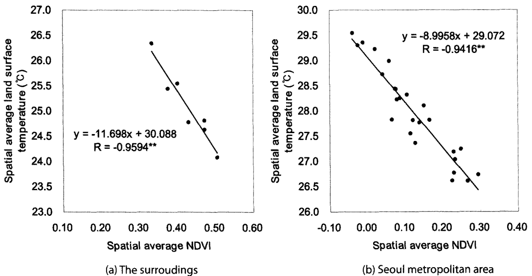
Figure 8. Associations between spatial average Normalized Difference Vegetation Index (NDVI) and land surface temperature derived from Landsat TM imagery (on July 26 in 1994) across the less urbanized areas in the outskirts (a) and across districts (Gus) within the Seoul metropolitan area (b). **: significant at the 99% level. Landsat TM 위성영상(1994년 7월 26일)에서 추출한 서울 도심내 각 구별(a) 또는 서울 외곽 도시화가 덜 된 지역(b)의 공간 평균 정규식생지수와 지표온도 간의 관련성.
