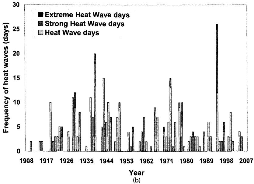
Figure 2. Inter-annual variations of annual average surface air temperature and annual total precipitation anomalies (a) and of annual total frequency of heat wave days, strong heat wave days and extreme heat wave days (b) in Seoul over the last 100 year period (1908-2007). Climatic anomalies are calculated based on the data for the entire 100 year period. 지난 100년(1907~2008) 동안의 서울의 연 평균 기온 및 연 총 강수량의 아노말리 (a)와 열파일, 강한 열파일, 극심한 열파일의 연 총 발생빈도(b)의 경년변화.
