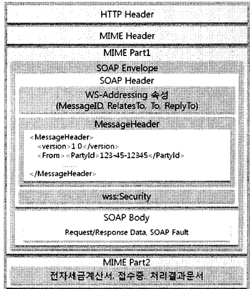
그림 2 전자세금계산서 전송을 위한 메시지 구조
