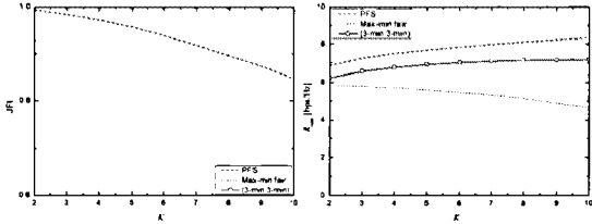
그림 3. 형평성을 추구하는 스케줄링 방법들의 형평성 및 총 전송률 합 성능.
