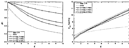
그림 1. 총 전송률 합을 추구하는 스케줄링 방법들의 형평성 및 총 전송률 합 성능
