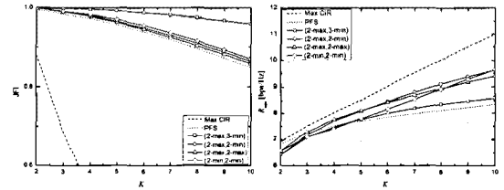
그림 2. PFS 방법에 준하는 형평성을 유지하면서 총 전송률 합을 추구하는 방법들의 형평성 및 총 전송률 합 성능
