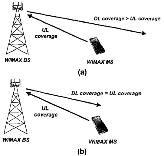
그림 1. Mobile WiMAX 기지국의 상/하향 커버리지 (a) 일반적인 기지국의 현재 상태 (b) 출력파워가 최적으로 설계된 상태
