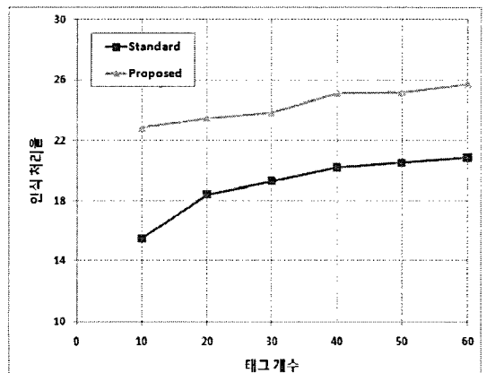
그림 8. 인식 처리율
