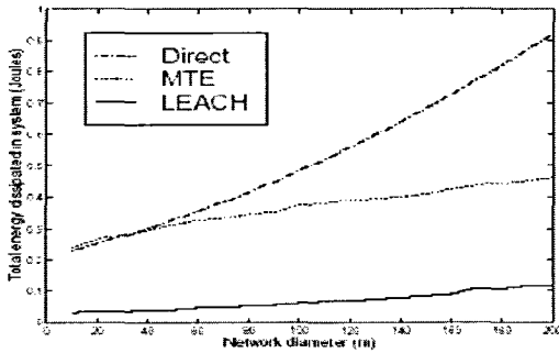
그림 12. LEACH 클러스터링 성능 Fig. 12. LEACH clustering efficiency
