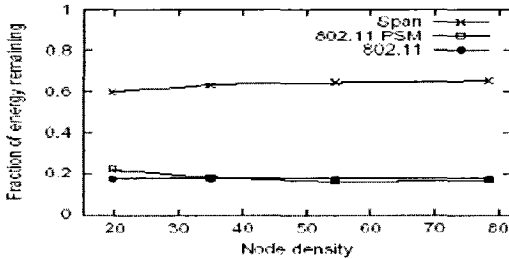
그림 11. SPAN 알고리즘의 성능 평가 Fig. 11. Efficiency valuation of SPAN algorithm
