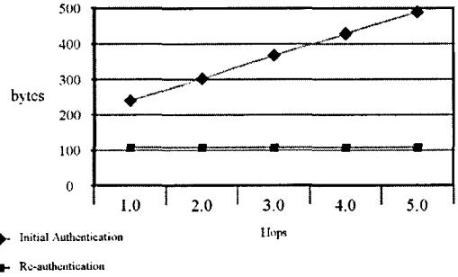
그림 5. 제안 기법의 초기 인증과 재인증 성능 비교
