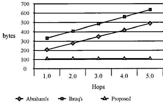
그림 6. 기존 기법과 재인증 성능 비교
