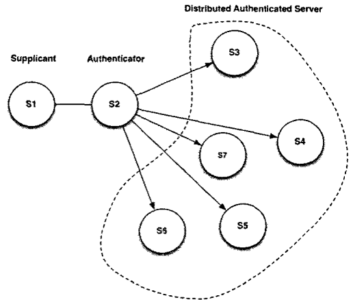
그림 2. Fantacci et al.의 센서 인증 기법 [1]
