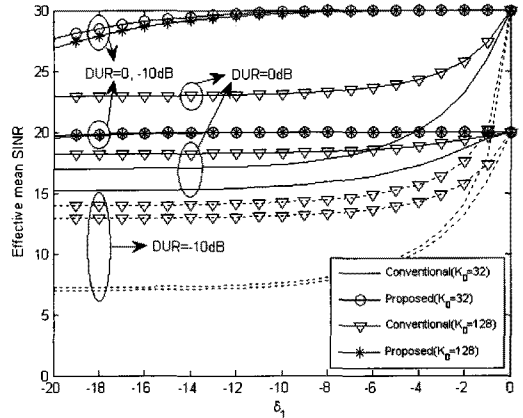
그림 6. Effective SINR
