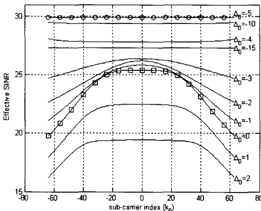
그림 5. Effective SINR ( N = 256 , G = 32 )
