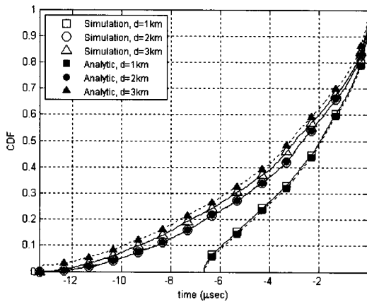
그림 2. TDoA의 CDF
