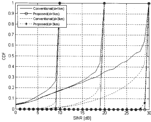
그림 7. SINR의 CDF
