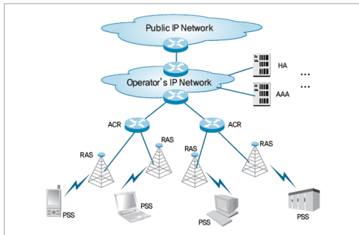
[그림 2] 와이브로망 구성도
