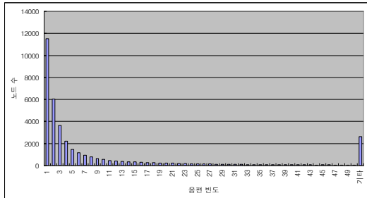
그림 4. 노드내 음편 수에 따른 히스토그램 Fig. 4. The histogram of the node numbers according to the segment numbers in each node
